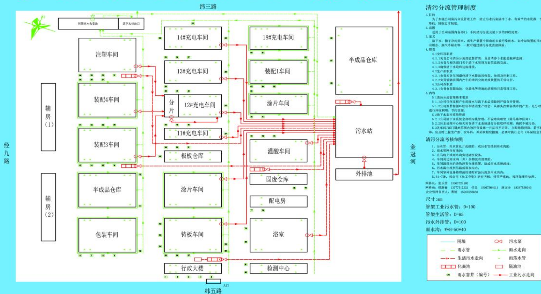
附图2 厂区雨污管线图
